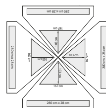
Nadruk na czterech owiewkach i czterech brytach zadaszenia
