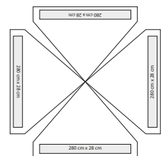
Nadruk na czterech owiewkach
