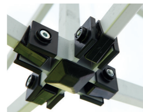
Verbindungen aus gegossenem Aluminium
